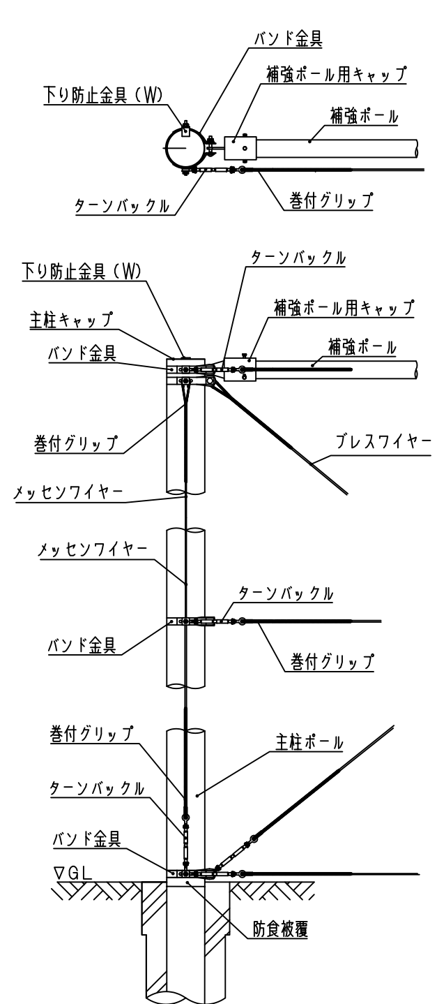
端末柱詳細図
