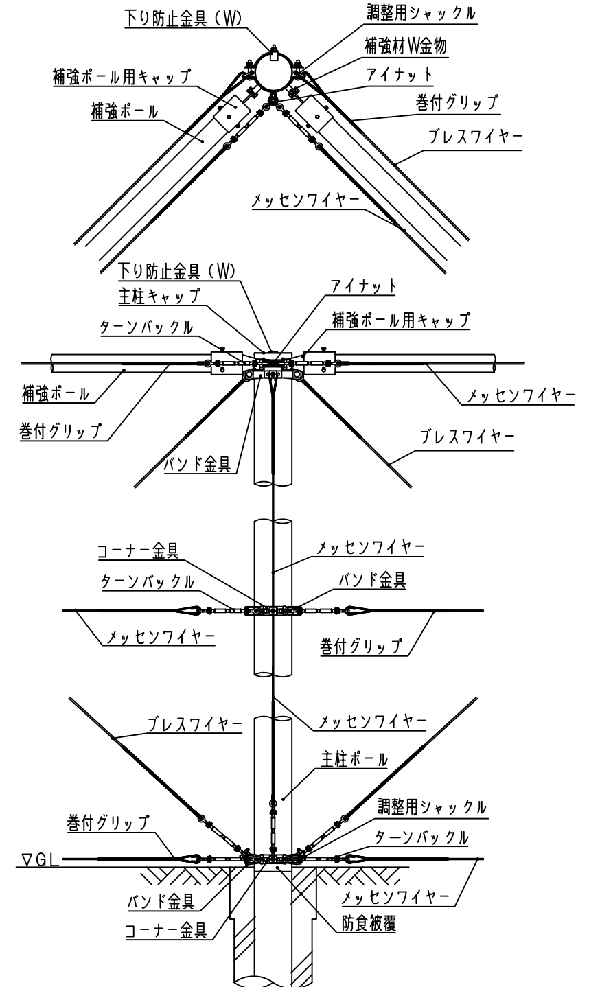
コーナー柱詳細図
