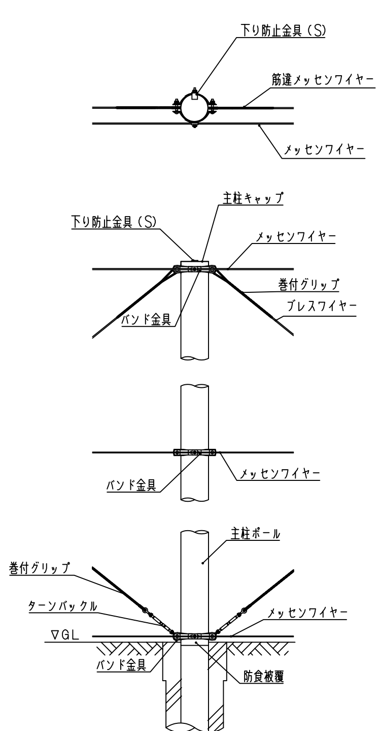
中間柱詳細図
